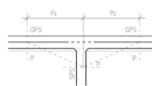
Slika 2a: Priključevanje brez priključnih zavijalnih lokov
